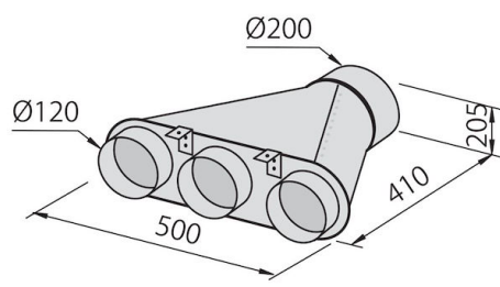
Collecteur pour 3 tubes 2524 000
